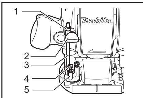
► 1. Apunador de profundidad 2. Tornillo 3. Tope de profundidad 4. Perno hexagonal de ajuste 5. Bloque de tope
