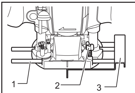
► 1. Guide bar 2. Clamp screw 3. Straight guide
